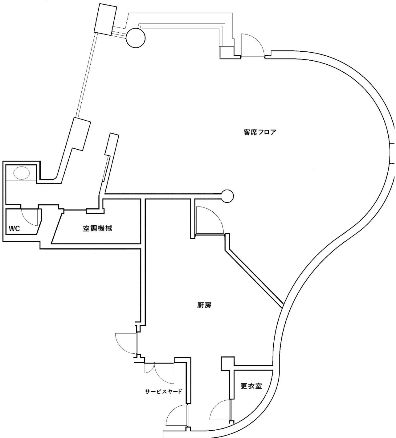
店舗平面図
